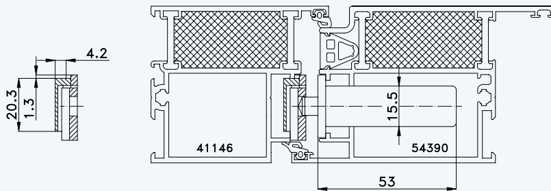
Situation Türfänger (bei Verriegelung mit Türwächter)
