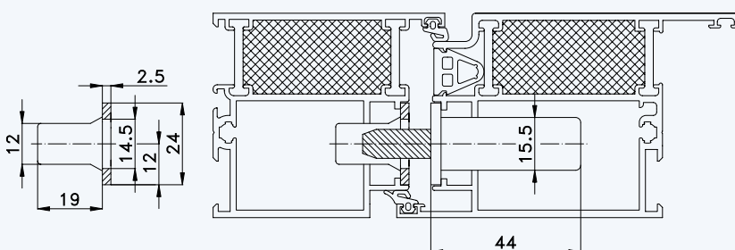
Situation Bolzen (bei Tresor-Bolzen-Verriegelung)
