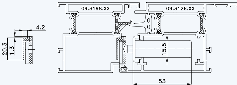
Situation Türfänger (bei Verriegelung mit Türwächter)
