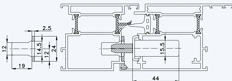
Situation Bolzen (bei Tresor-Bolzen-Verriegelung)
