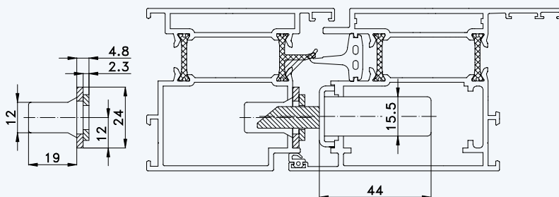
Situation Massivschwenkriegel (bei Automatik-Verriegelung)
