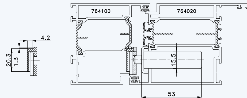
Situation Türfänger (bei Verriegelung mit Türwächter)
