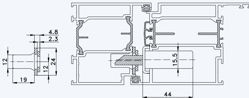
Situation Massivschwenkriegel (bei Automatik-Verriegelung)
