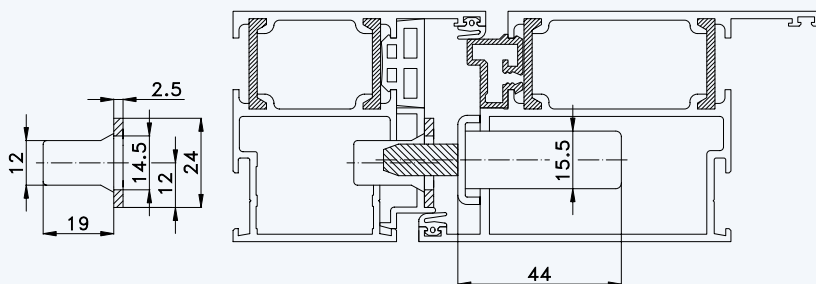
Situation Bolzen (bei Tresor-Bolzen-Verriegelung)
