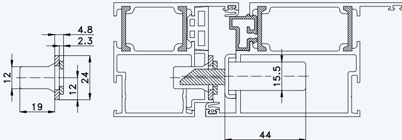
Situation Massivschwenkriegel (bei Automatik-Verriegelung)
